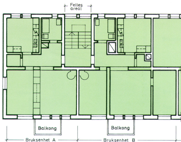
Fig. 15 Bruksareal i bolighus. Figuren viser to bruksenheter. Trappehuset utgjør en felles del. Bruksareal er egnet til å angi størrelse på del av bygning
